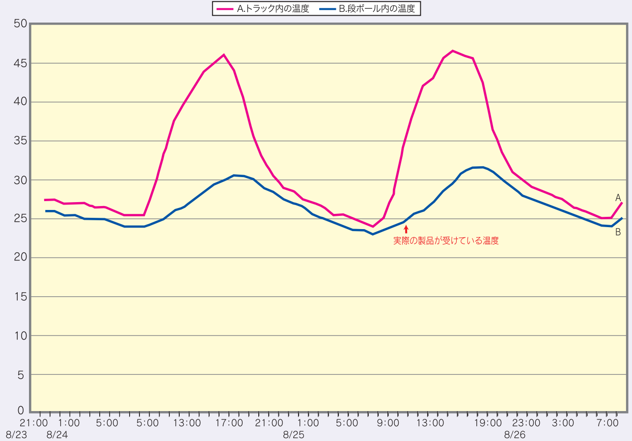
2008年8月24~26日 関東から関西へのトラック輸送中の温度変化
