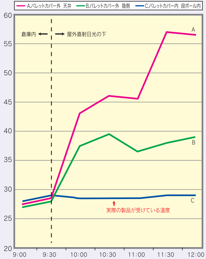
2008年8月9日 弊社屋外実験にて直射日光及びトラック内の温度実験
